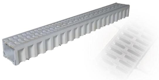
CANAL E GRELHA PP 1000x130x80
